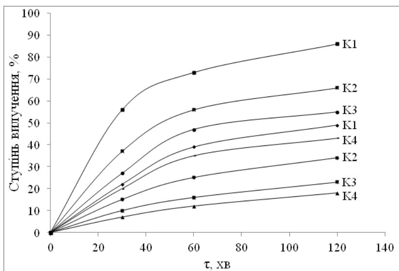
Рис. 1. Залежність ступеня вилучення фосфат-іонів від тривалості сорбції для зразків K1-K4, синтезованих прожарюванням при 300 °С і 350 °С.
