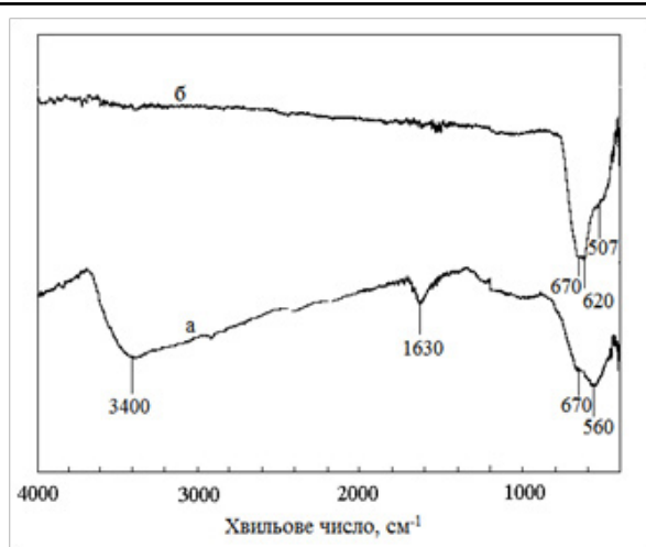
Рис. 2. ІЧ-спектри зразків \text{SnO}_2 : а — термооброблений при T=723 К, б — термооброблений при T=1023 К.
