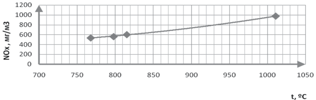
Рис. 1. Залежність вмісту NO x у продуктах згоряння від температури спалювання довгополуменового вугілля
