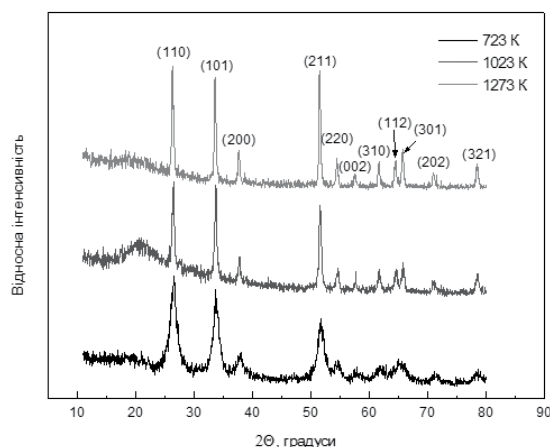
Рис. 1. Дифрактограми зразків \text{SnO}_2 .
