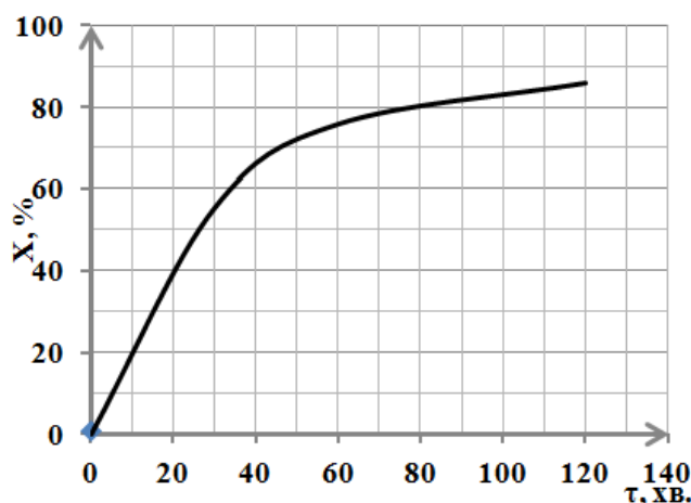
Рис. 2. Залежність ступеня вилучення фосфат-іонів із водного розчину сорбентом від тривалості процесу.
